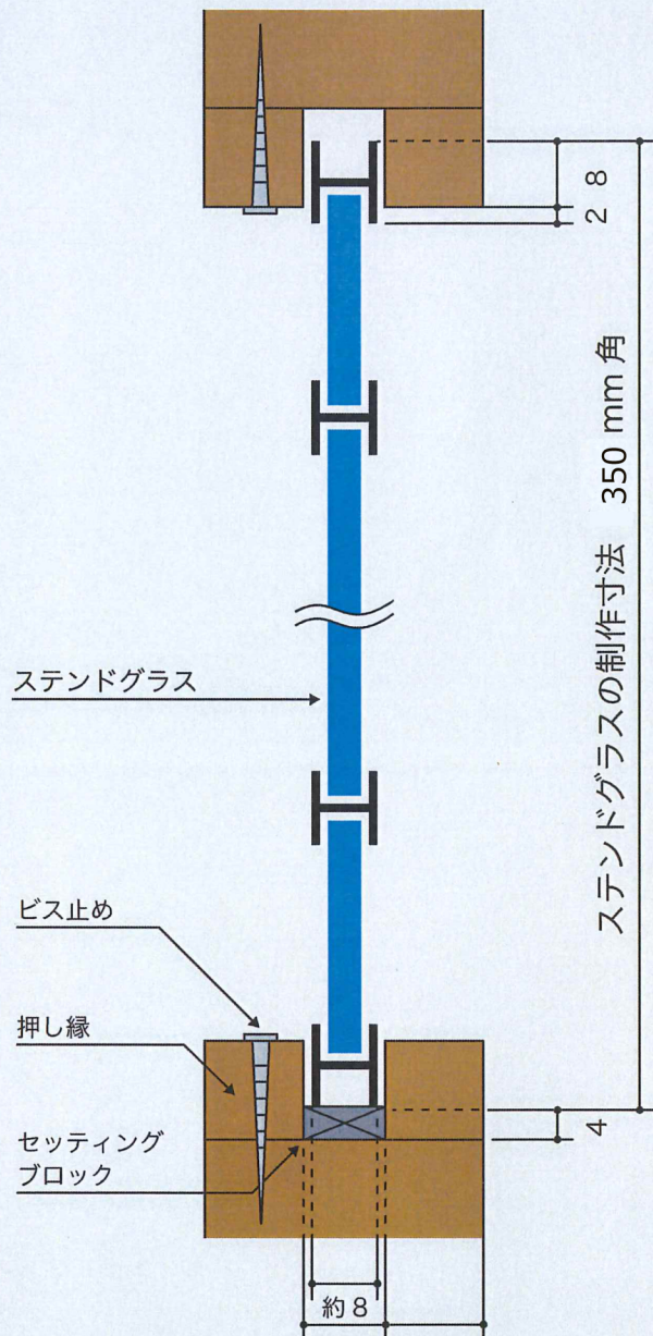
縦横共通 取付断面図 (mm)
