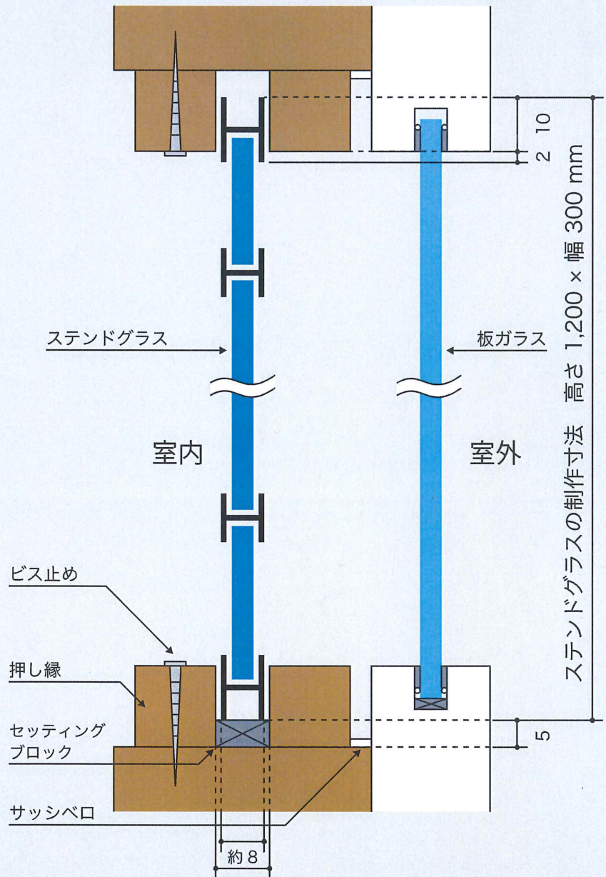
縦横共通 取付断面図 (mm)
